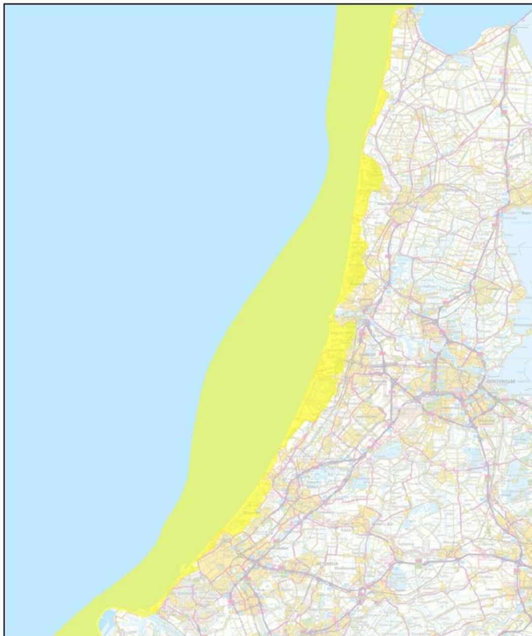
Detailkaart 3 kustfundament
