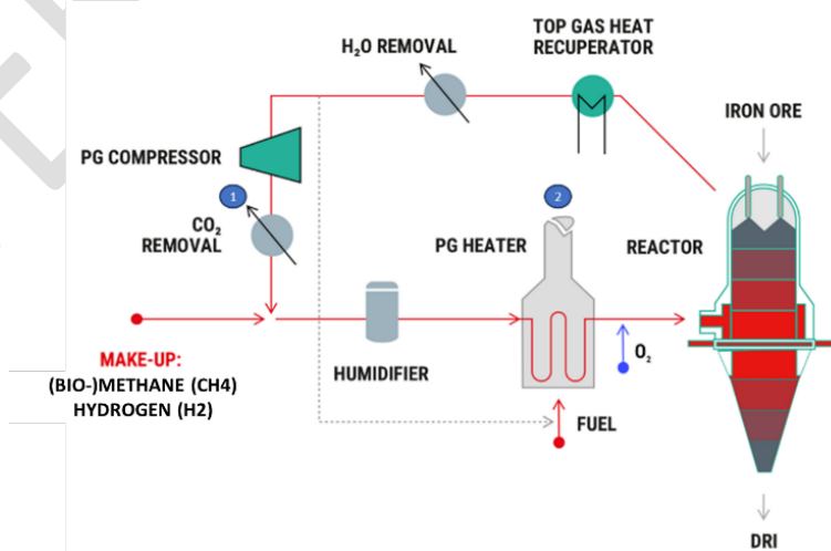
Afb. 2: Stroomschema DRP met emissiepunten 1 en 2 (Energiron® DRP-technologie)
