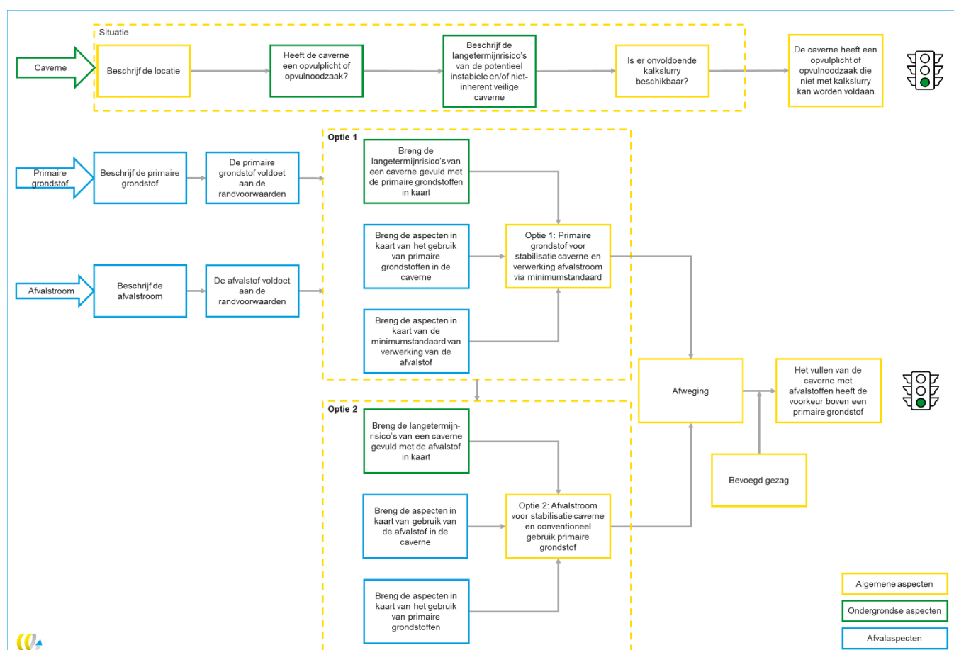
Figuur 3 – Schematische weergave van het afwegingskader voor het gebruik van afvalstoffen om een zoutcaveerne inherent veilig te maken. Voor een grotere versie, zie Bijlage C.
