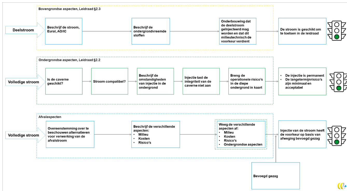
Figuur 4 - Stappenplan voor afwegingskader injectie productieafval in zoutcavernes (voor een grotere versie, zie Bijlage C)
