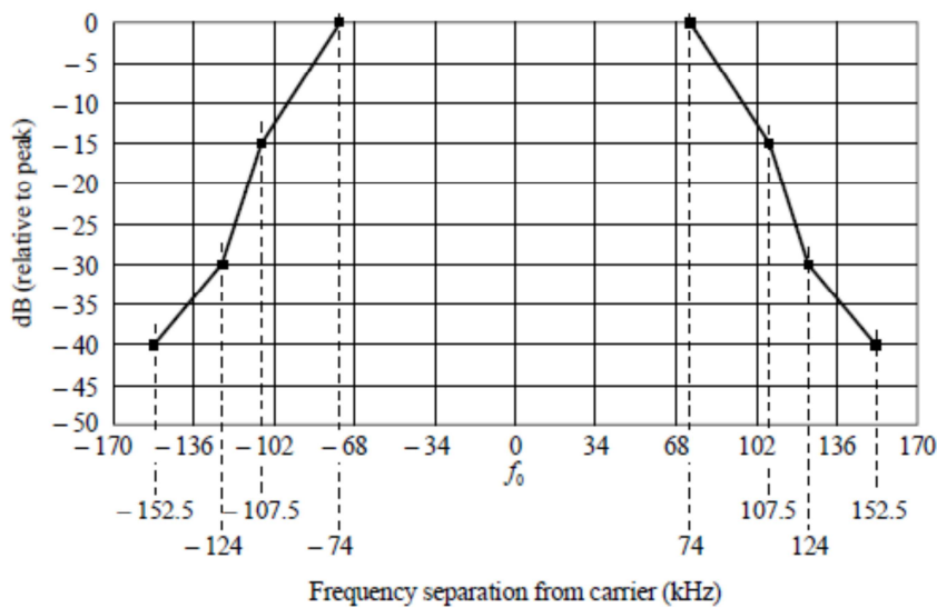
Figuur 1: Spectrummasker voor FM-uitzendingen. Bron: ITU-R SM 1268-3
